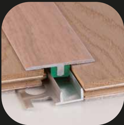
Perfil de expansión + guía Base de aluminio
